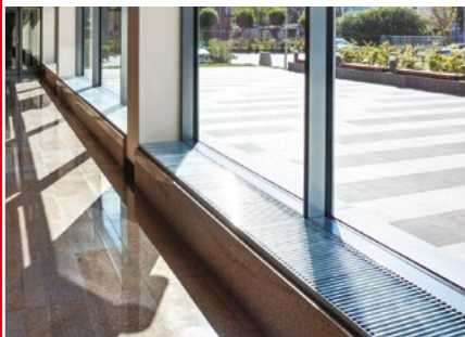
VK15 BODENKONVEKTOR MIT NATÜRLICHER KONVEKTION
