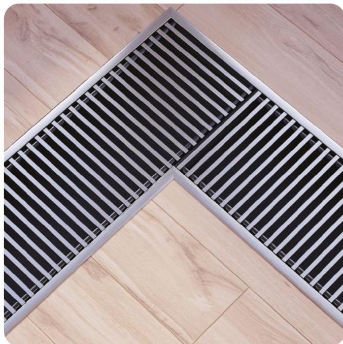
| Eck Bodenkonvektoren mit Quer-Roste und F-Rahmen.
