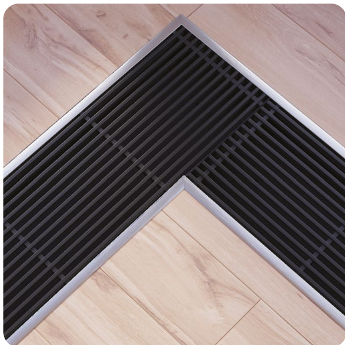
| Eck Bodenkonvektoren mit Längsroste und F-Rahmen.
