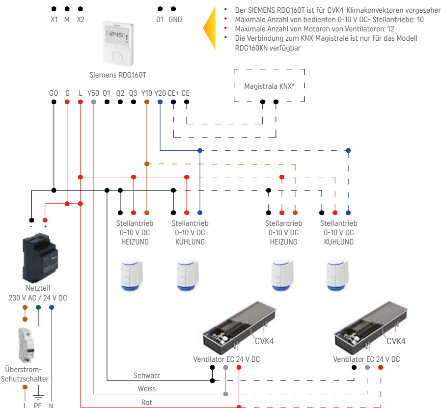
Ein Beispielschlussplan eines oder mehrerer CVK4 Klimakonvektoren
